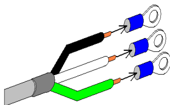
図 2-5. 電源ケーブル加工図
