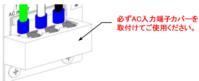
図 2-1. 1200W タイプ電源コード接続
