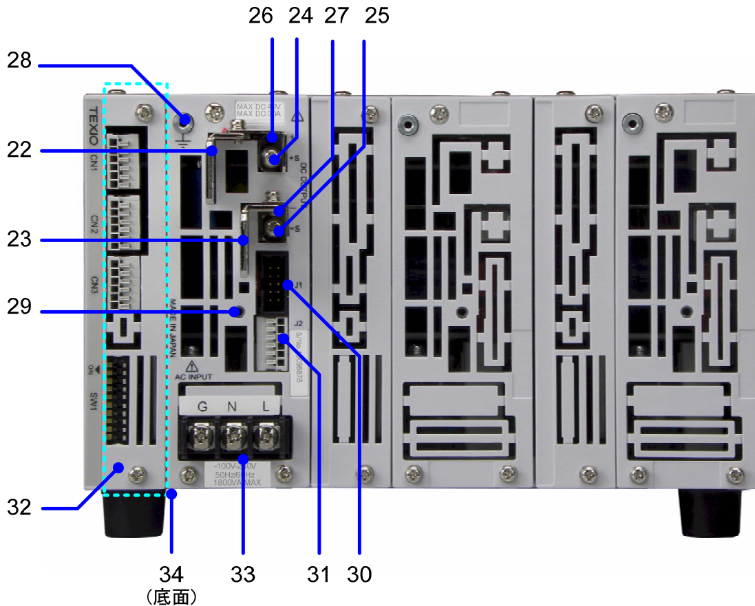
図 3-3 背面パネル
