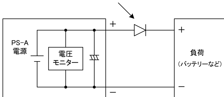
図 4-1 エネルギーを持った負荷の接続
