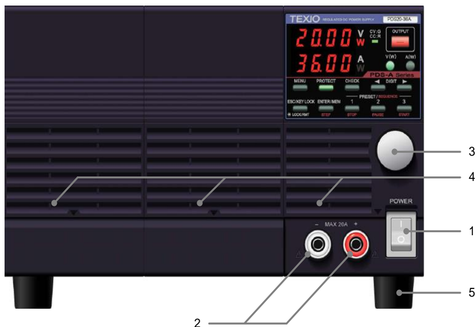
図 3-1 前面パネル (図は PDS20-36A です)
