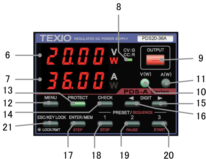
図 3-2 操作パネル部
